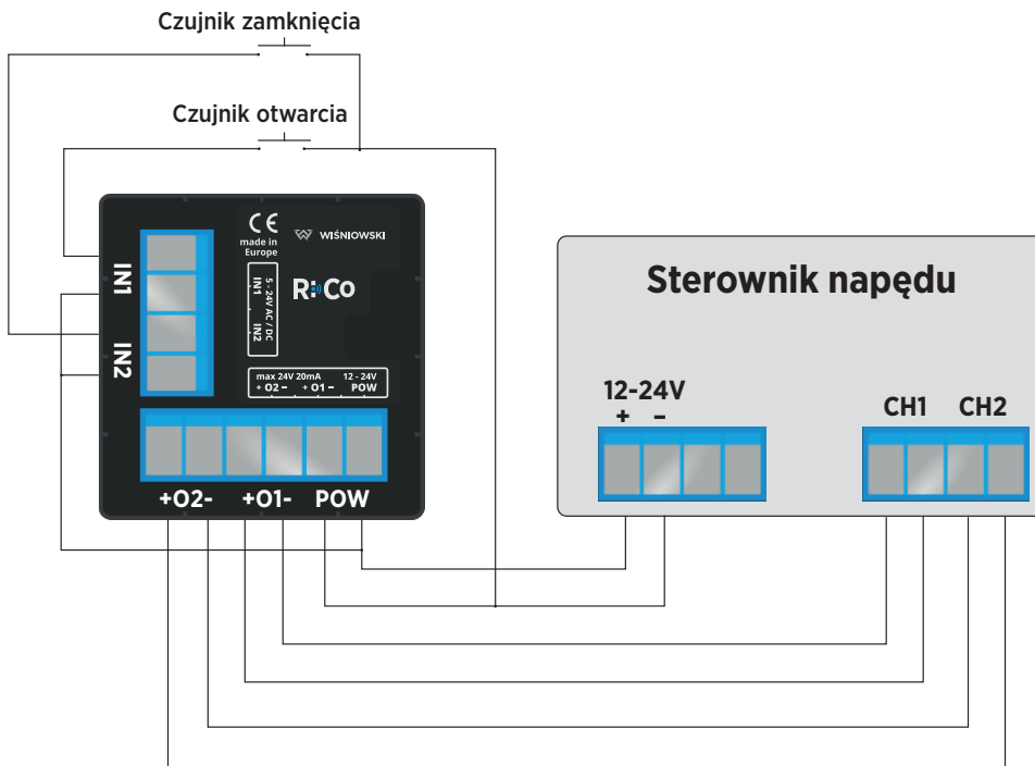
Rysunek 1 Podłączenie Ri-Co do sterownika napędu
